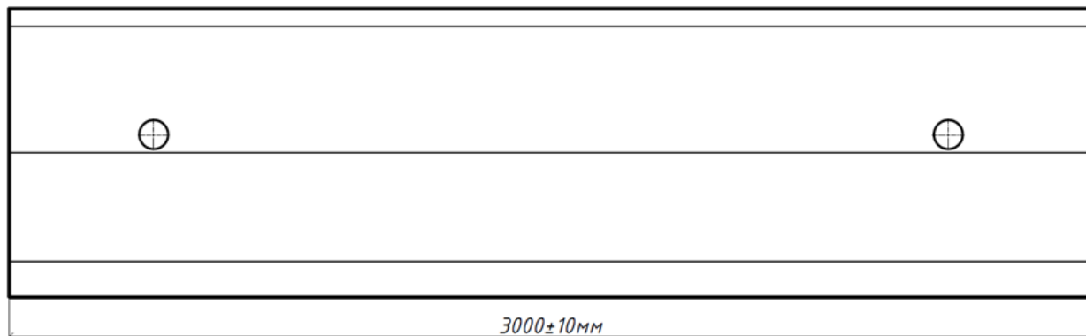
Блок ограждения железобетонный вид спереди Темірбетонды қоршау блогы алдыңғы көрініс
