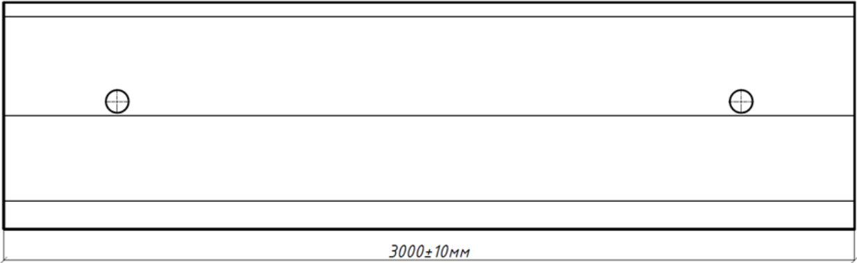
Блок ограждения железобетонный вид спереди Темірбетонды қоршау блогы алдыңғы көрініс
