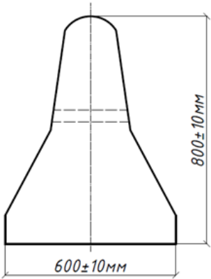
Блок ограждения железобетонный вид спереди Темірбетонды қоршау блогы алдыңғы көрініс
