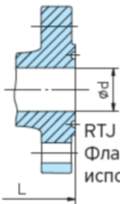
RF Фланцевое
