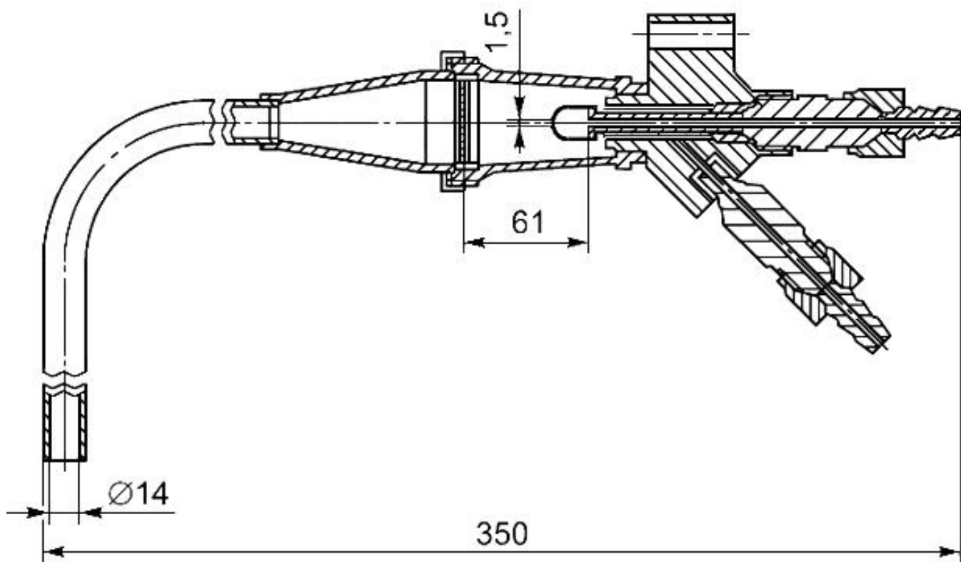
б - схема генератора пены
