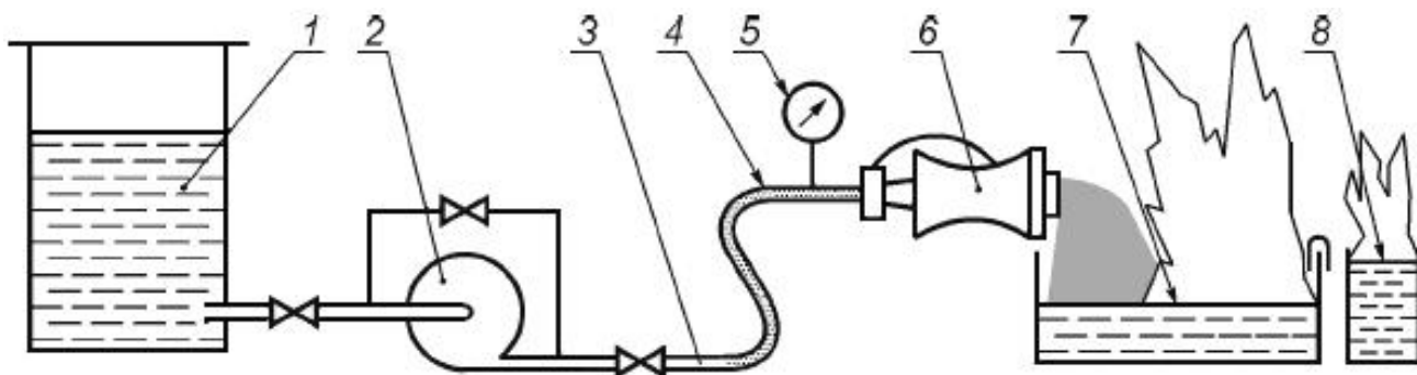
Рисунок 7 - Схема установки для тушения пеной средней кратности
