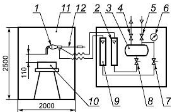
Рисунок 6 - Схема установки для тушения пеной средней кратности (стендовая методика)
