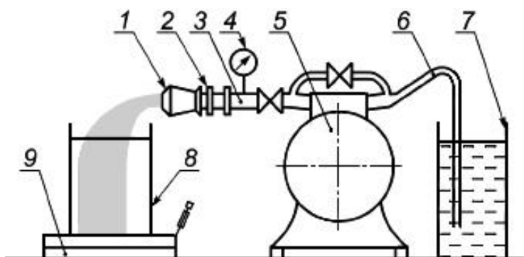
Рисунок 1 - Схема установки для определения кратности и показателя устойчивости пены
