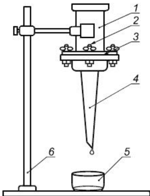
Рисунок 14 - Устройство для определения показателя смачивающей способности
