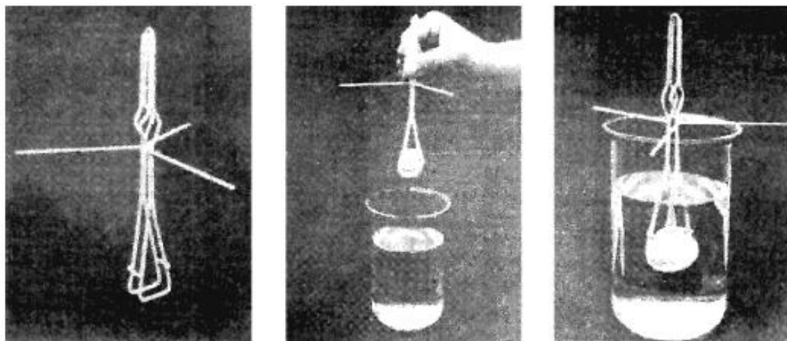
а - общий вид зажимного приспособления б - образец, помещенный в зажимы приспособления в - образец, погруженный в рабочий раствор
