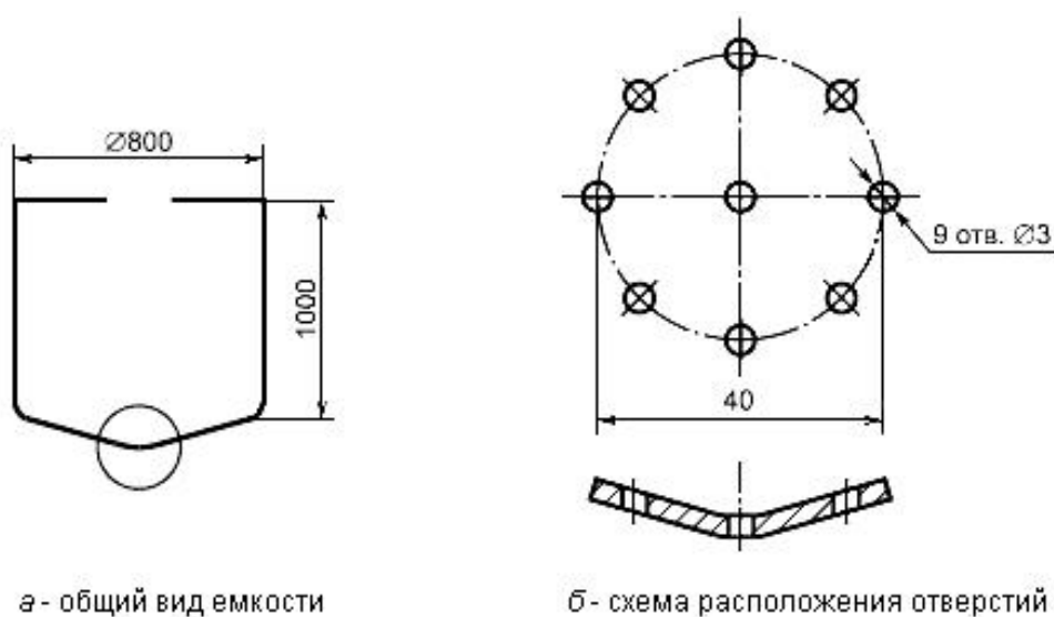
Рисунок 5 - Емкость для сбора пены
