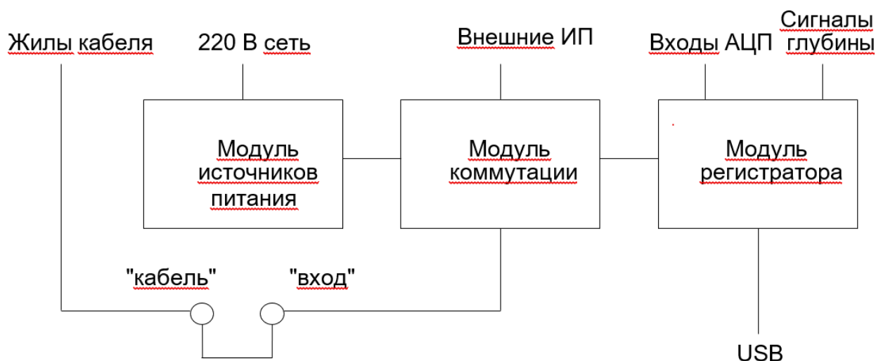
Рисунок 3. Структурная схема.
