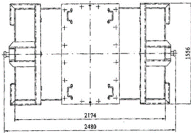
Рисунок. Транспортный упаковочный комплект ТУК-118
