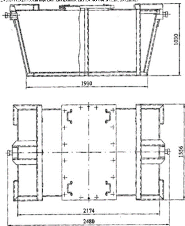
Рисунок. Транспортный упаковочный комплект ТУК-118
