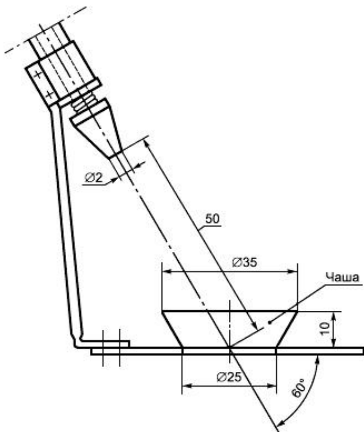
Рисунок 4 - Разбрызгиватель
