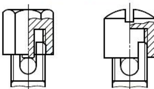
ж) Закрытые резьбовые выводы с прижимной гайкой
