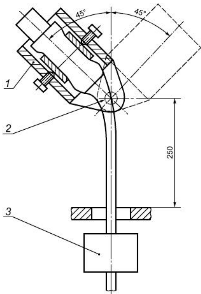
Рисунок 9 - Устройство для испытания на изгиб
