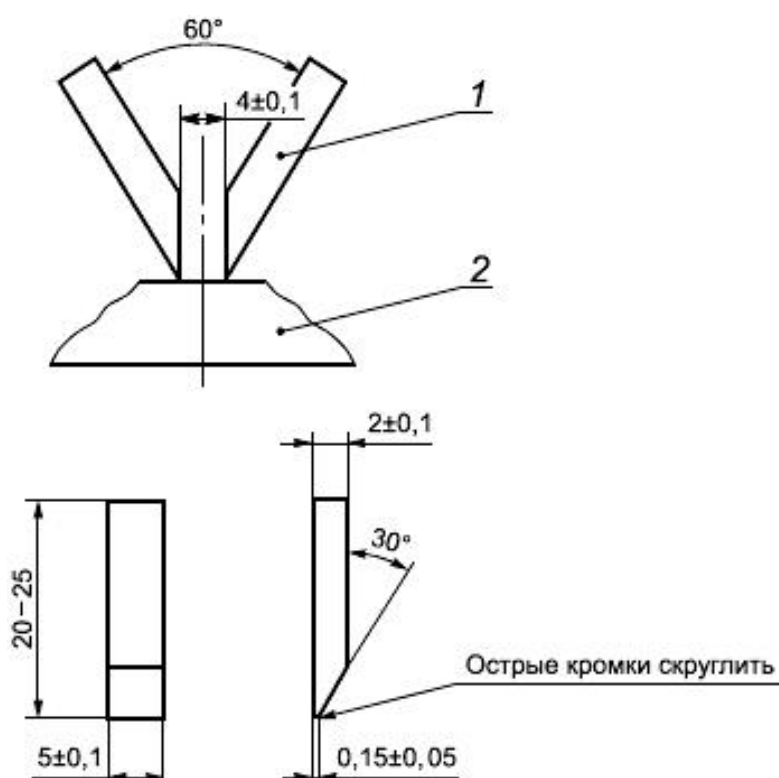
Рисунок 12 - Конструкция и положение на образце электродов для испытаний на стойкость к скользящим токам
