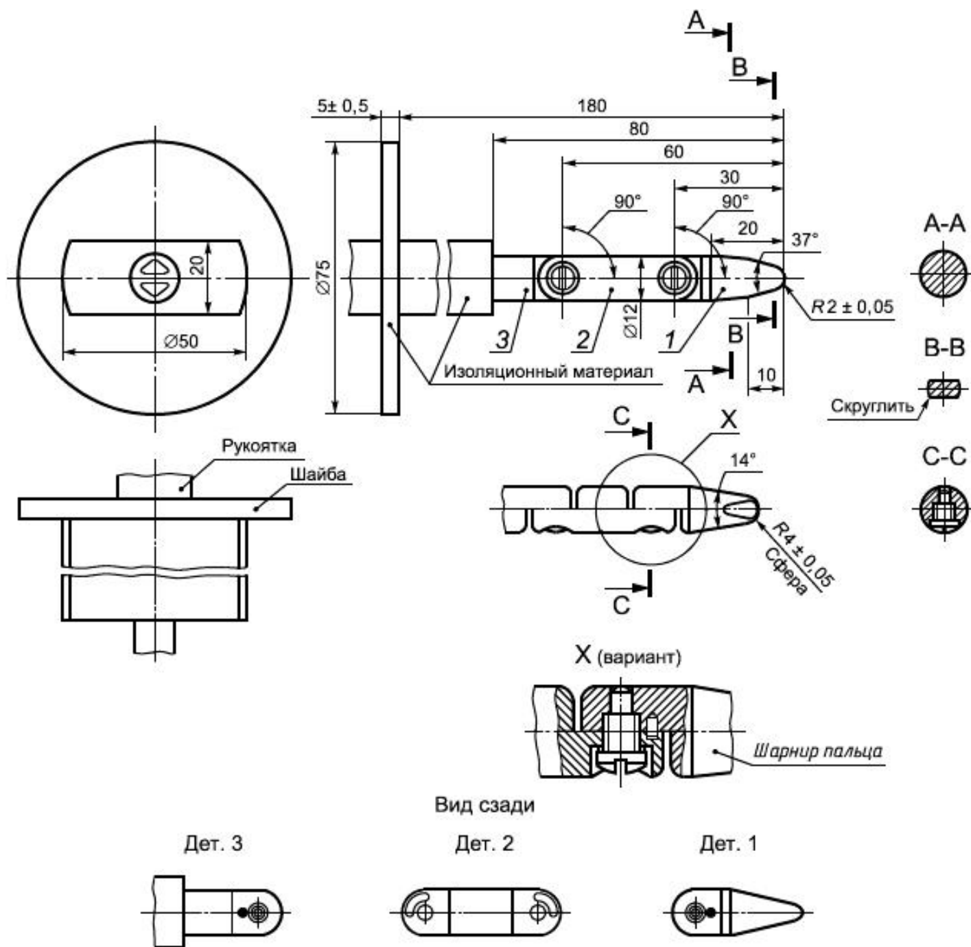
Рисунок 2 - Стандартный испытательный палец
