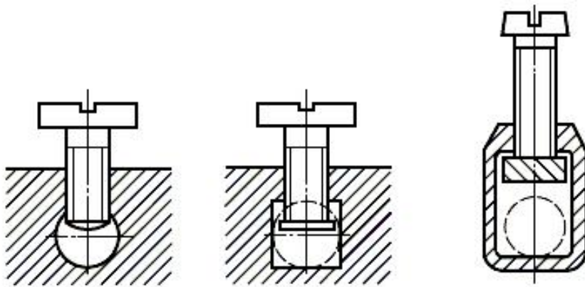
а) Столбчатые выводы
