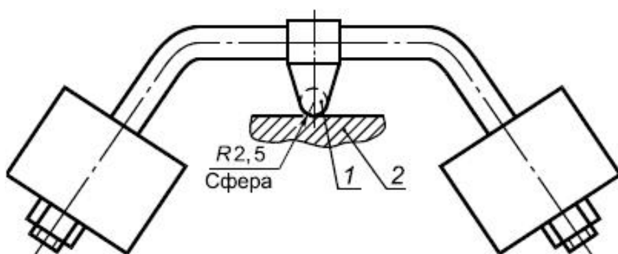
Рисунок 10 - Установка для испытаний давлением шарика
