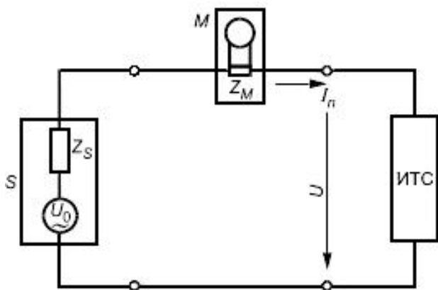
Рисунок А.1 - Схема измерений для однофазных ТС
