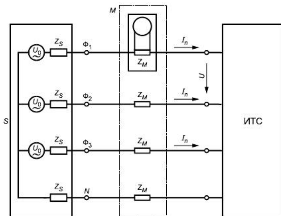
Рисунок А.2 - Схема измерений для трехфазных ТС
