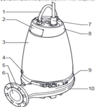
Рис. 1 Насос SE
