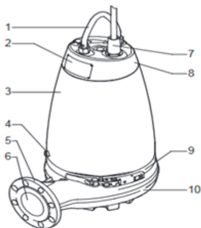
Рис. 1 Насос SE
