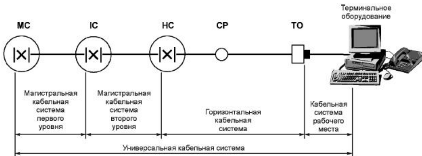
Рисунок 3 - Подсистемы СКС
