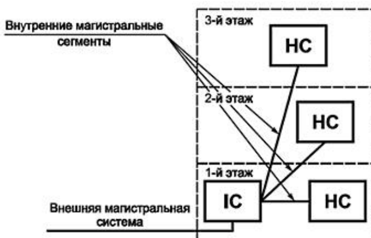
Рисунок 26. - Внутренняя магистральная кабельная подсистема (магистральная подсистема здания)
