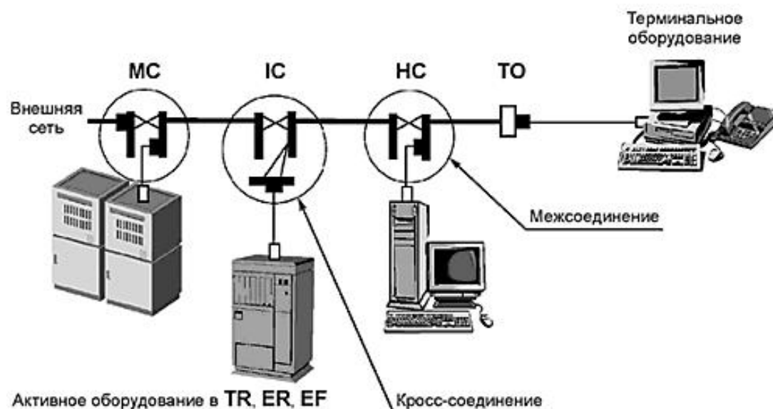
Рисунок 7. - Интерфейсы кабельной системы
