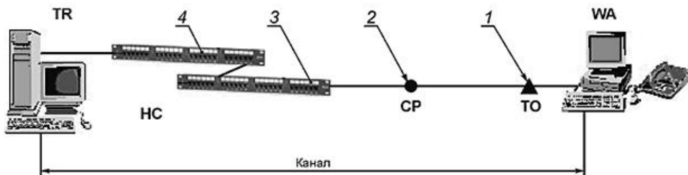
Рисунок 18. - Модель канала горизонтальной кабельной подсистемы с четырьмя точками коммутации
