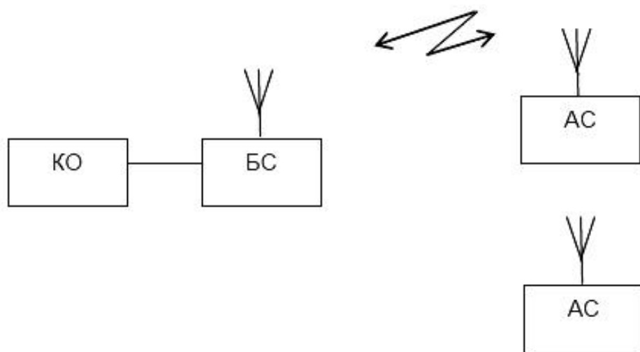
Рисунок 4.1 - Структурная схема организации однозоновой сети подвижной радиосвязи
