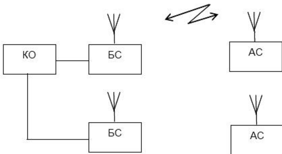
Рисунок 4.2 - Структурная схема организации многозоновой сети подвижной радиосвязи
