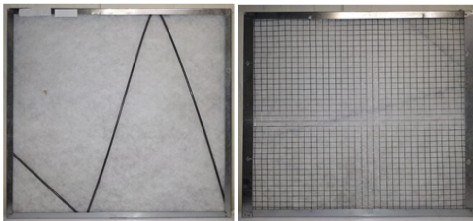
Рисунок 1 – внешний вид префильтра
