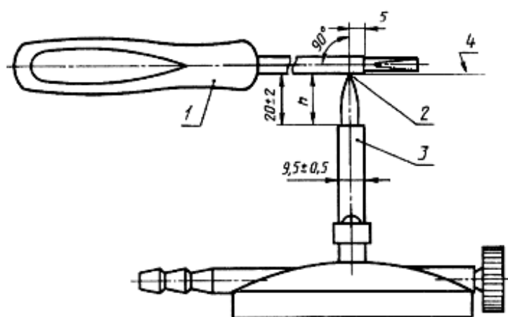
Рисунок 11 - Оборудование для испытания на воспламеняемость
