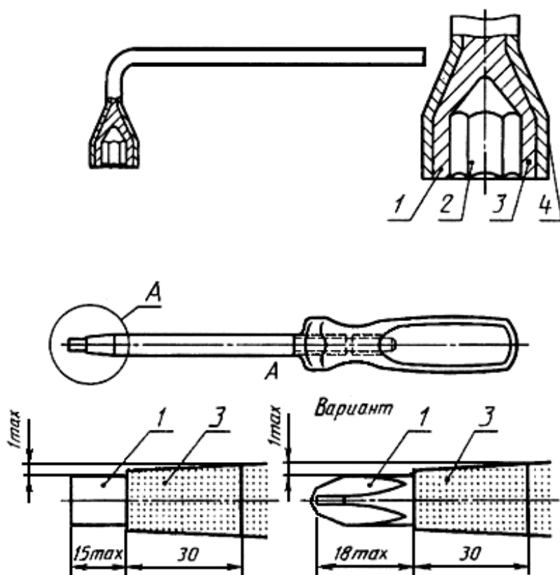
Рисунок 1 - Типы изоляции инструментов
