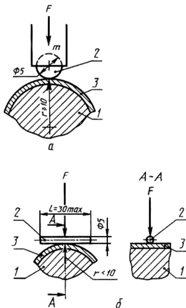
Рисунок 7 - Механическое испытание изоляции инструмента
