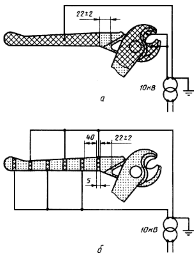
Рисунок 6 - Оборудование для электрического испытания изолирующих инструментов
