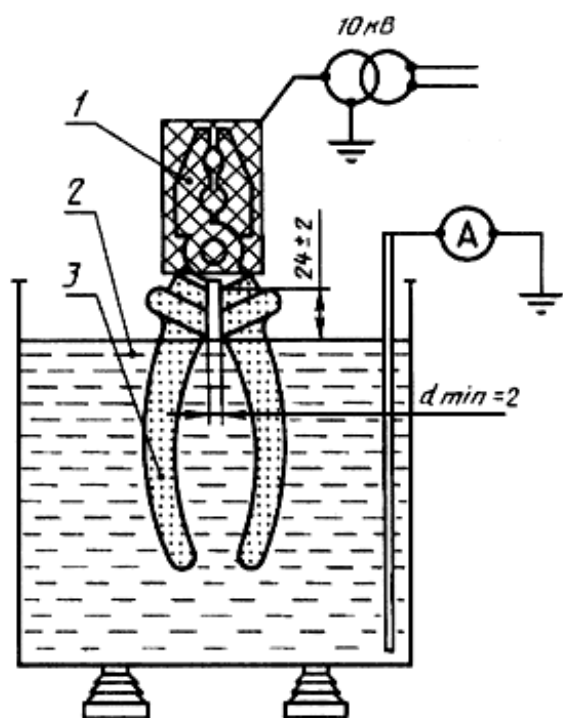
Рисунок 5 - Оборудование для электрического испытания изолированных инструментов
