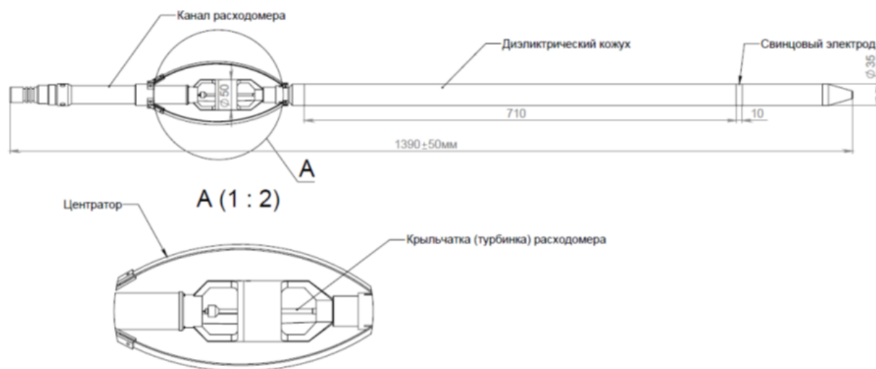
Рис. №1 «Расходомер совмещённый с прибором токового каротажа»
