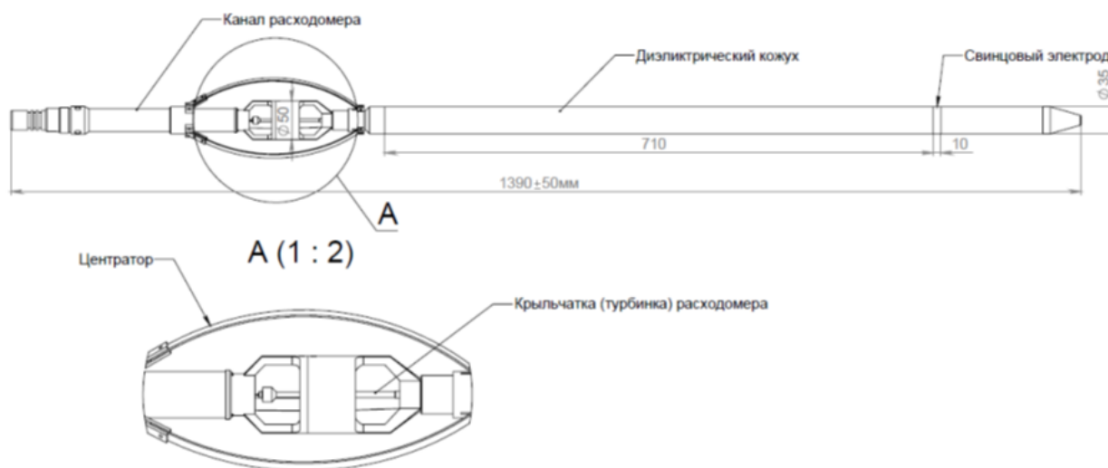
№1 сурет "Ағымдық қаротаж аспабымен біріктірілген шығын өлшегіш"
