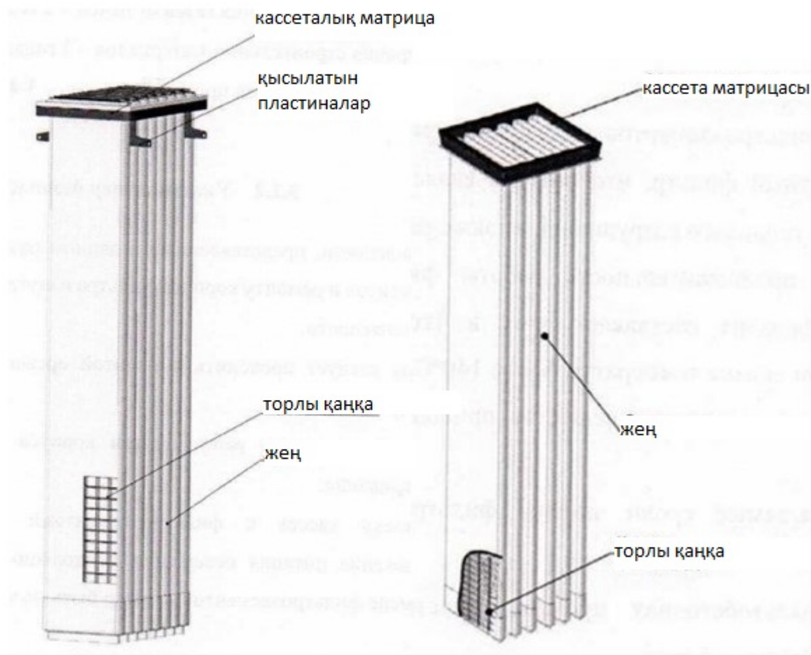
1-сурет. Жең сүзгілерінің жиынтығы
