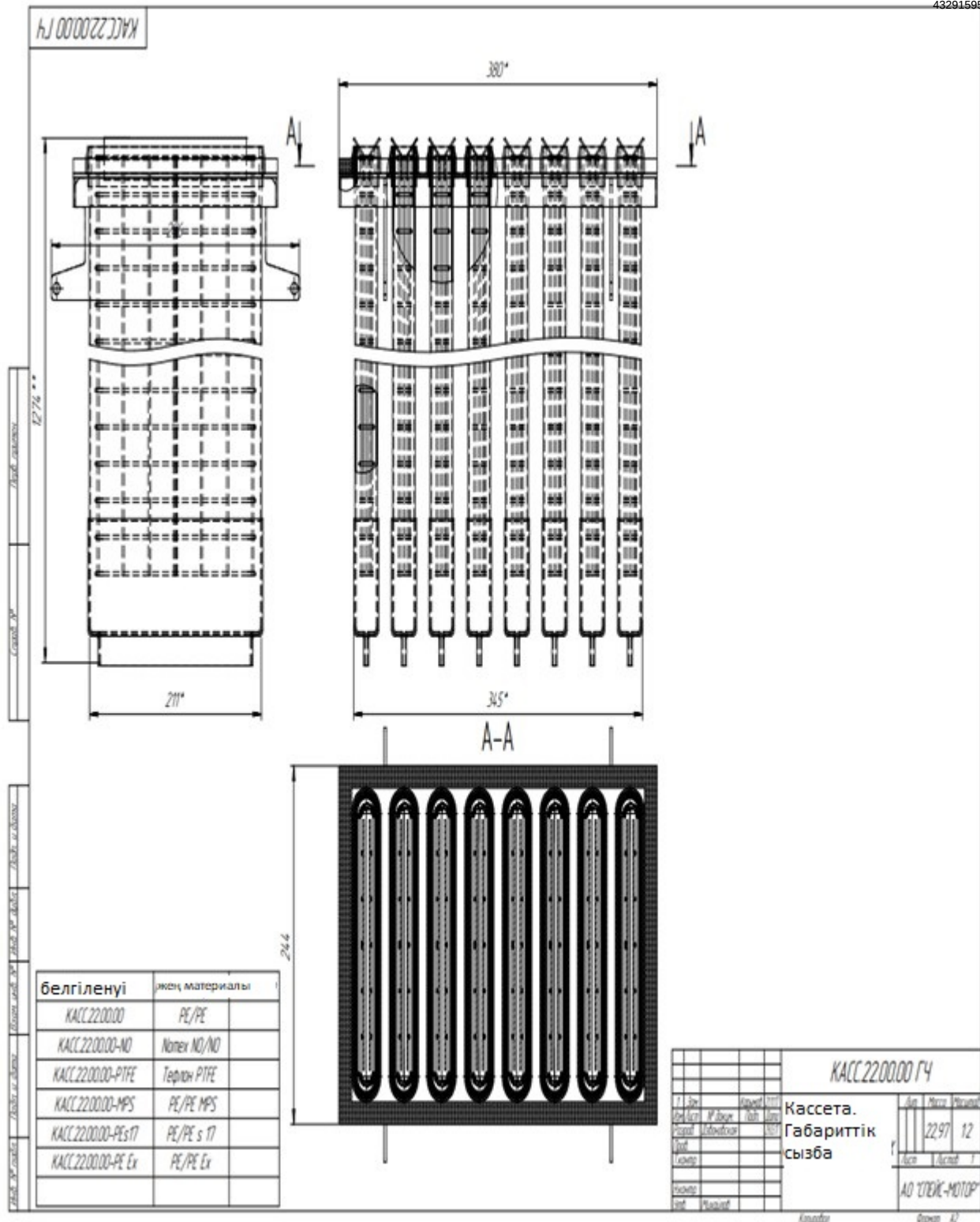
2-сурет. Габариттік сызба
