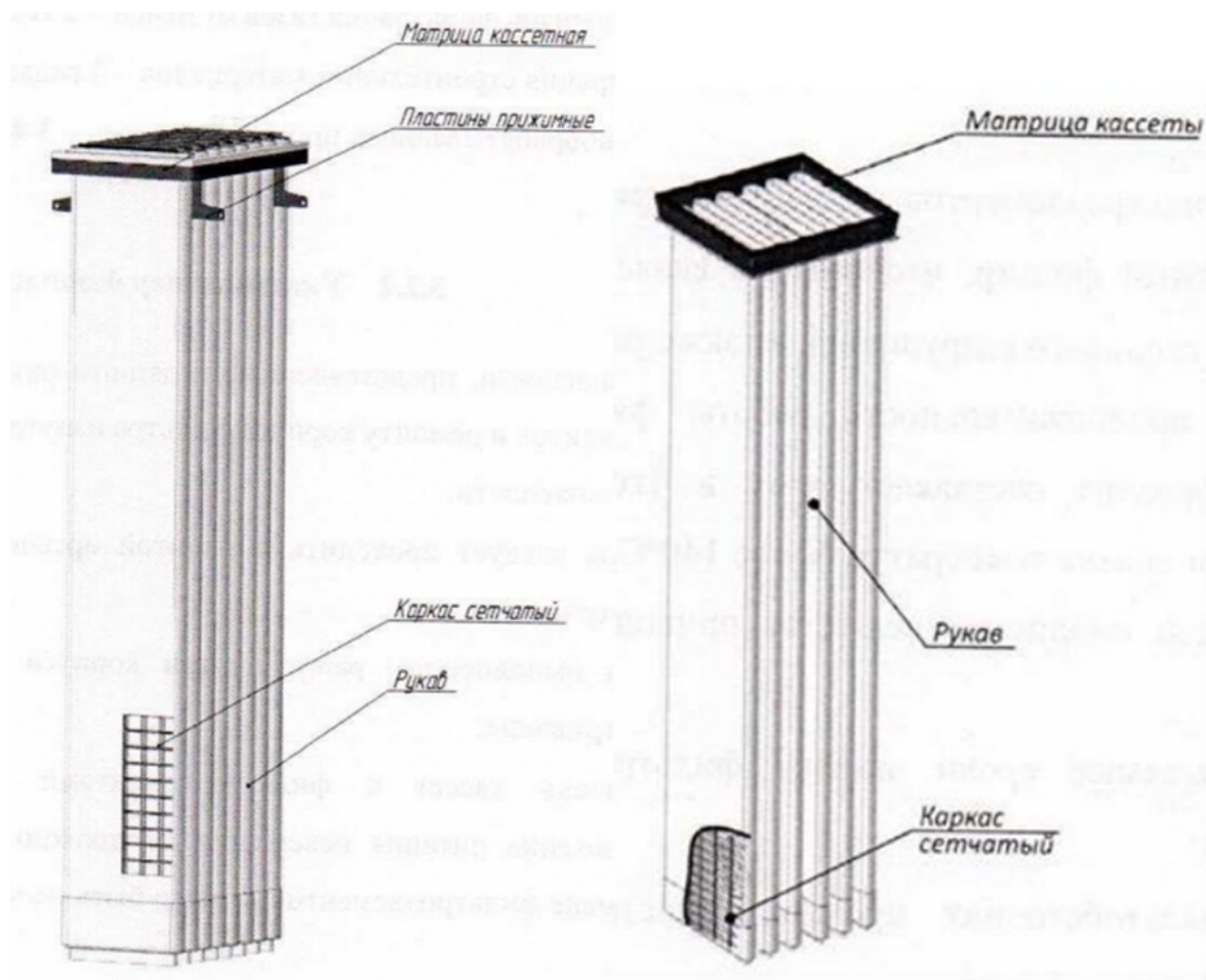
Рисунок 1. Комплект рукавных фильтров
